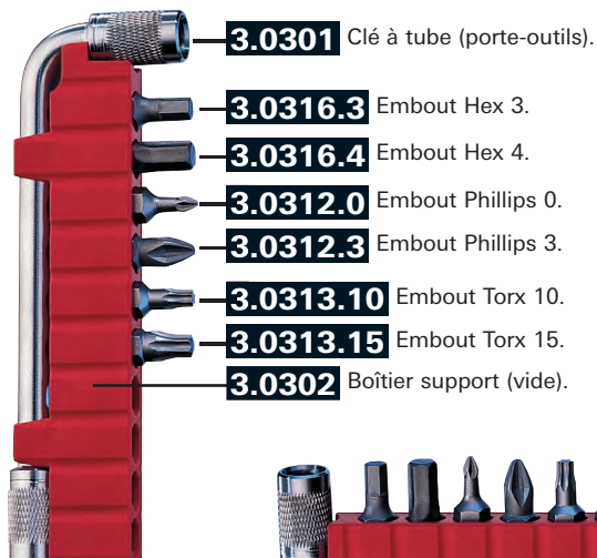
3.0303 Boîtier support complet (clé à tube porte-outils et 6 embouts).
