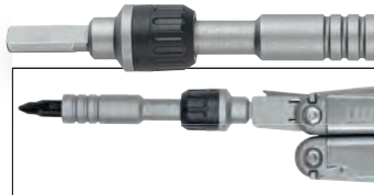
931030 RATCHET DRIVER Tournevis à cliquet avec porte-embout magnétique. Longueur : 8,3 cm. Compatible avec les pinces Wave +, Charge + TTI, Skeletool et Surge et les embouts du kit réf. 931014.
